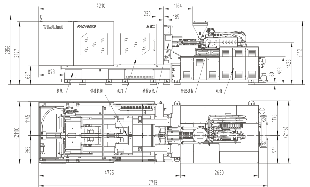
PAC460K3外形图
