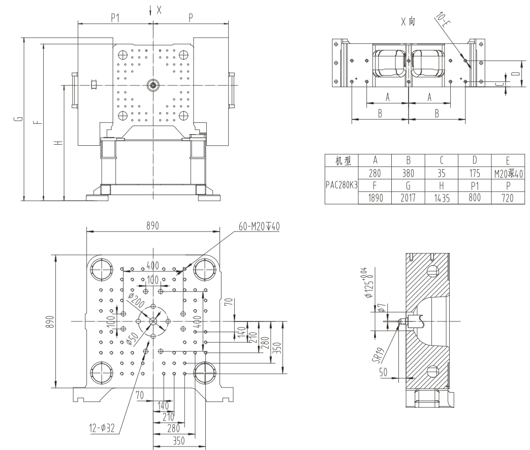
PAC280K3外形图
