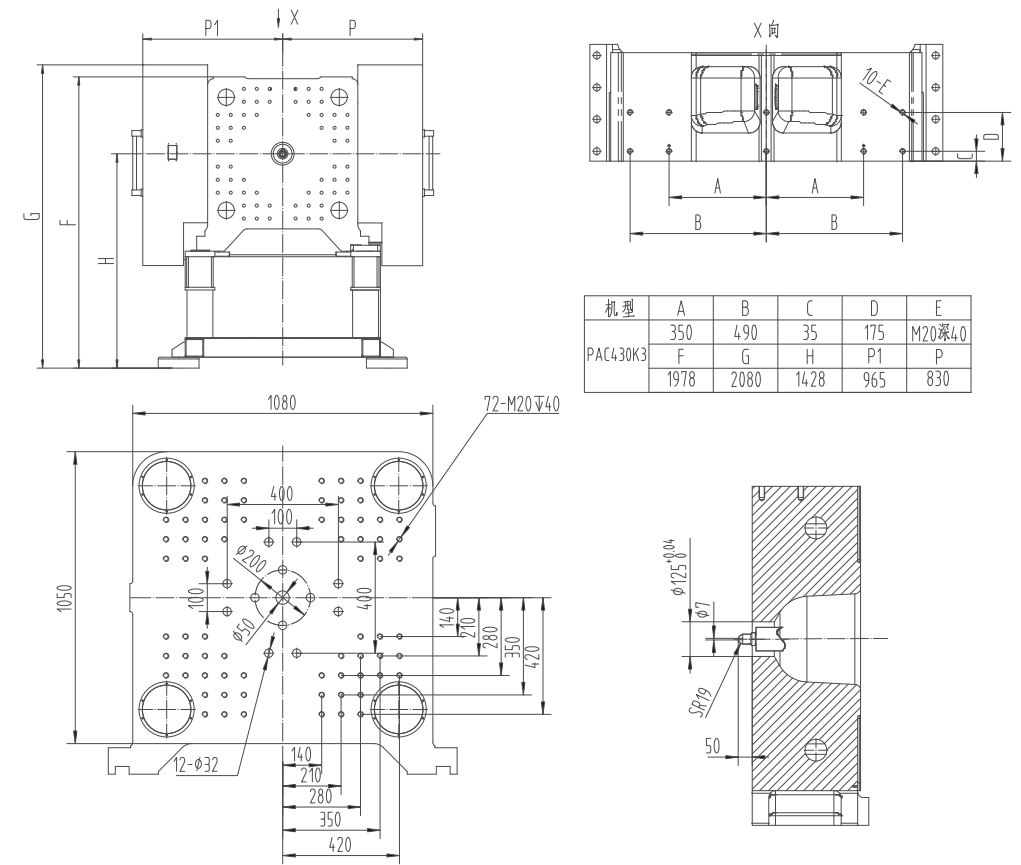
PAC430K3外形图
