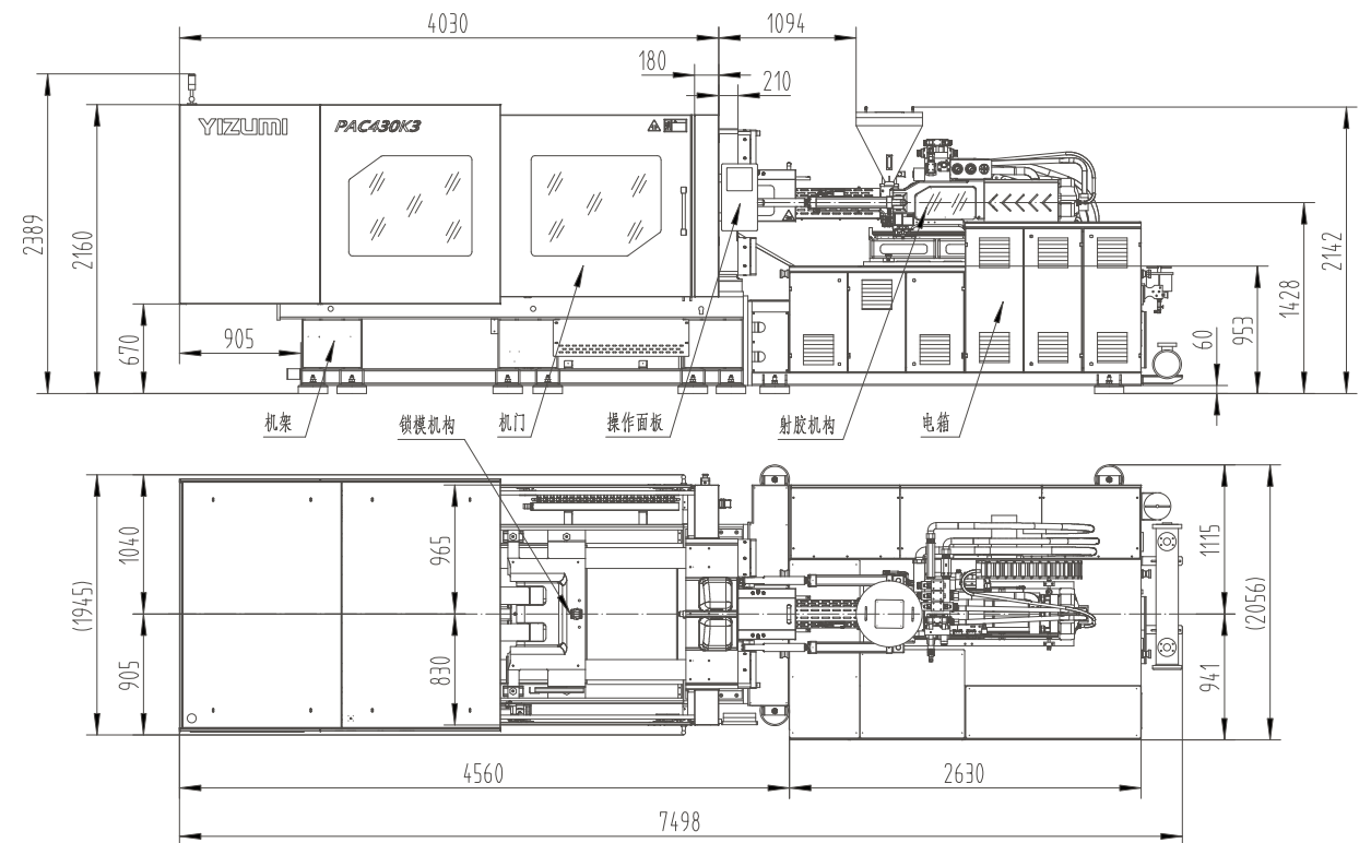
PAC430K3外形图
