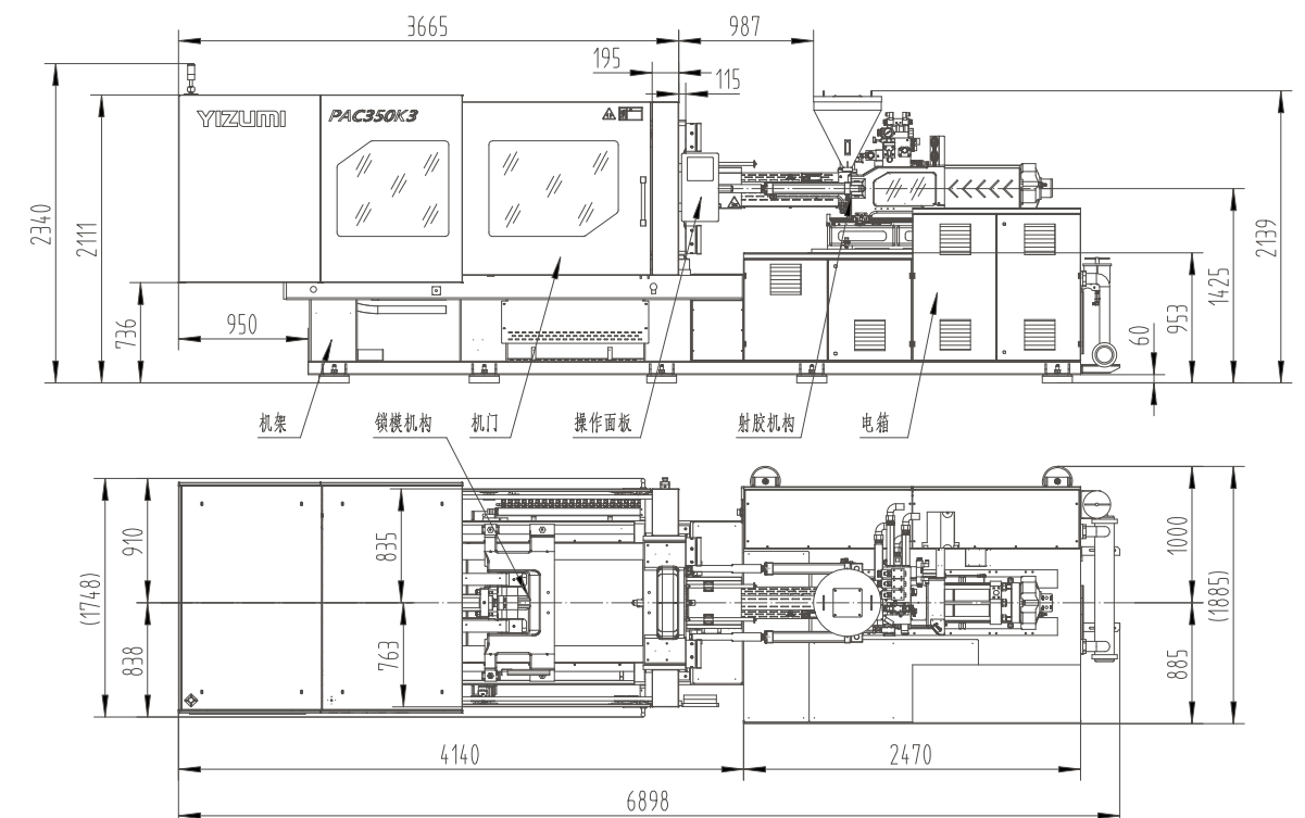
PAC350K3外形图
