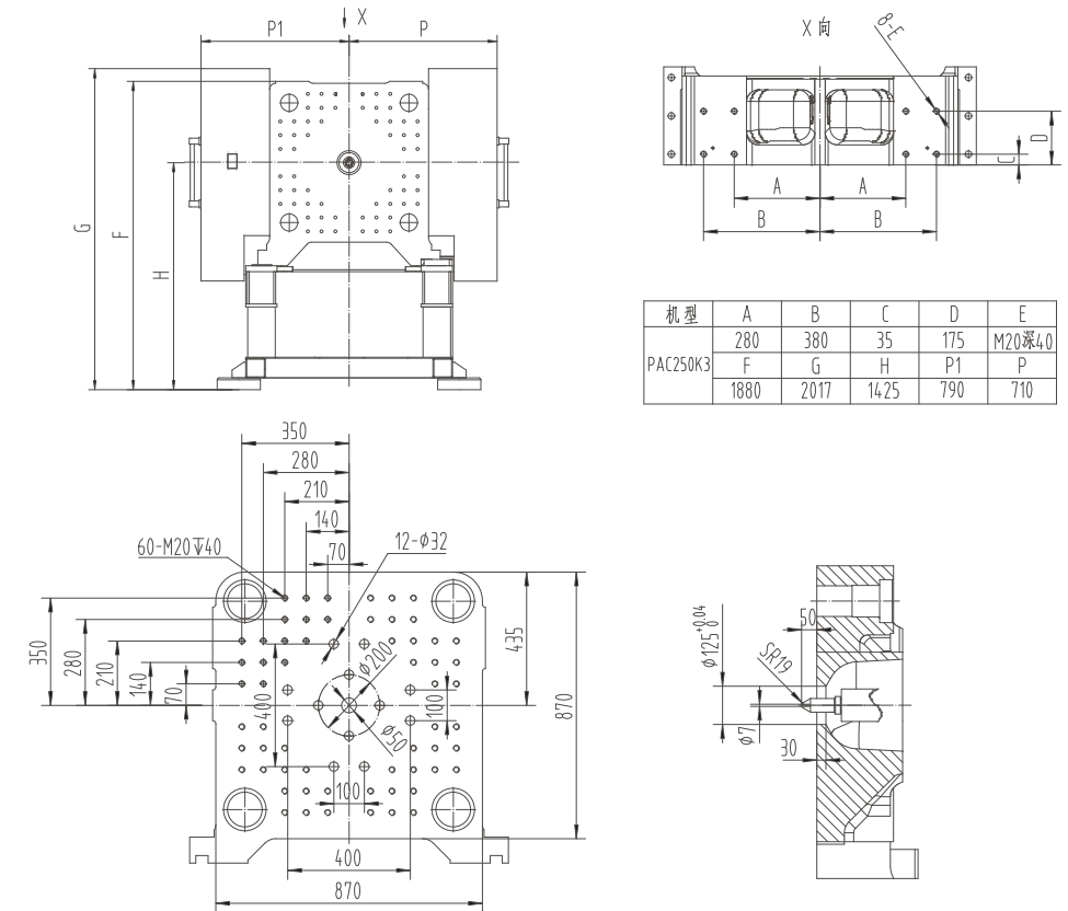
PAC250K3外形图
