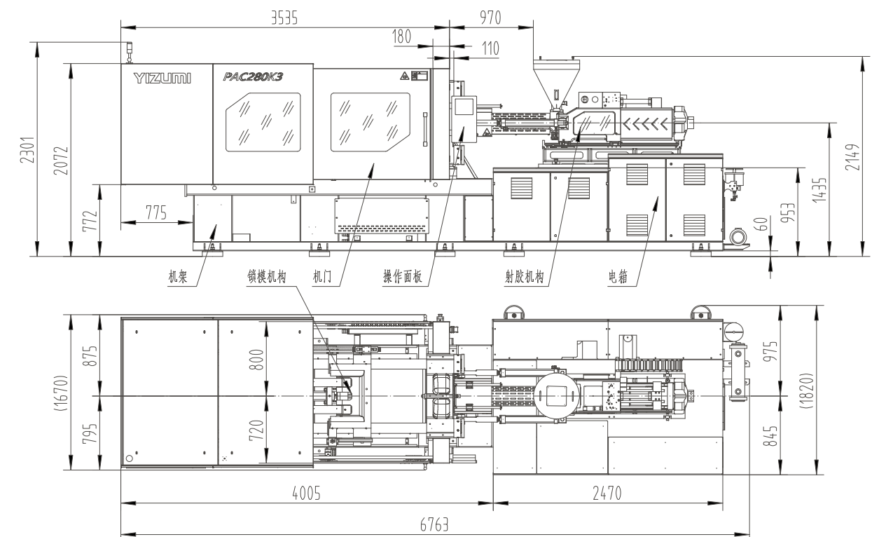
PAC280K3外形图
