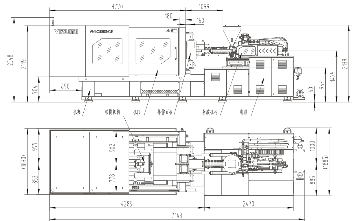
PAC380K3外形图
