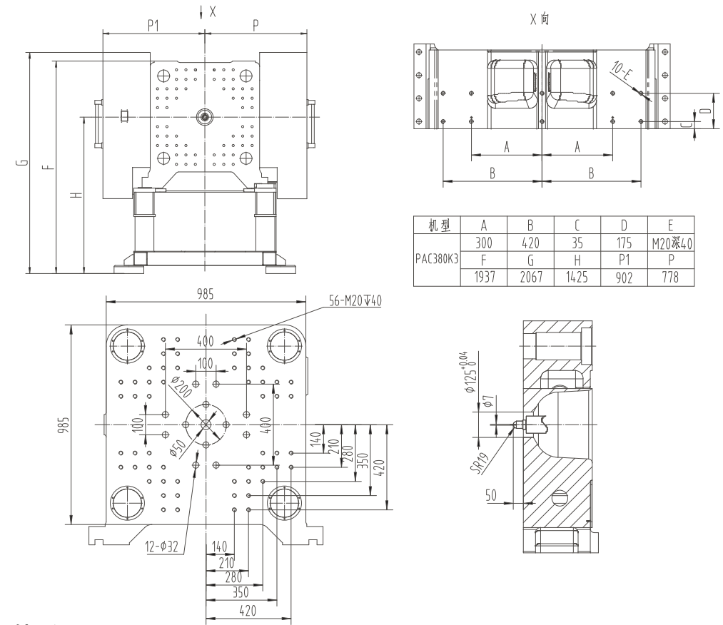
PAC380K3外形图
