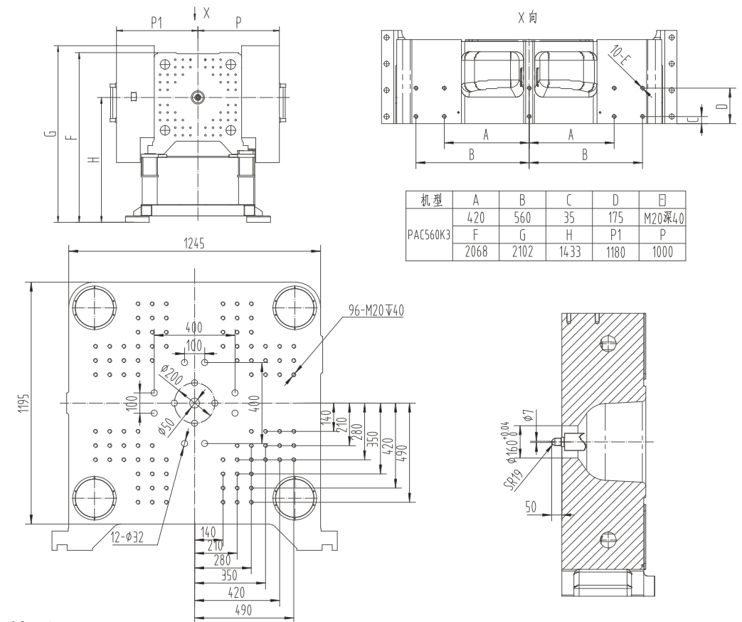
PAC560K3外形图
