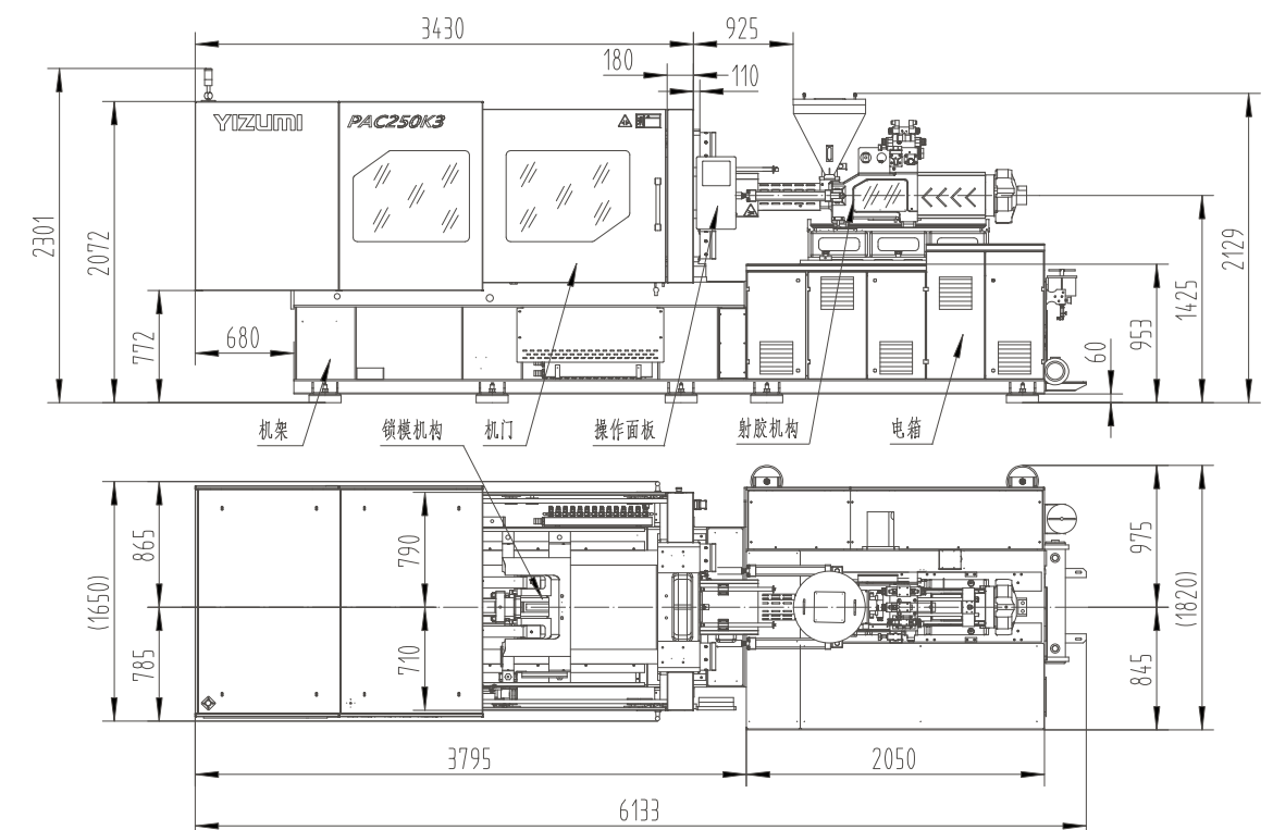
PAC250K3外形图
