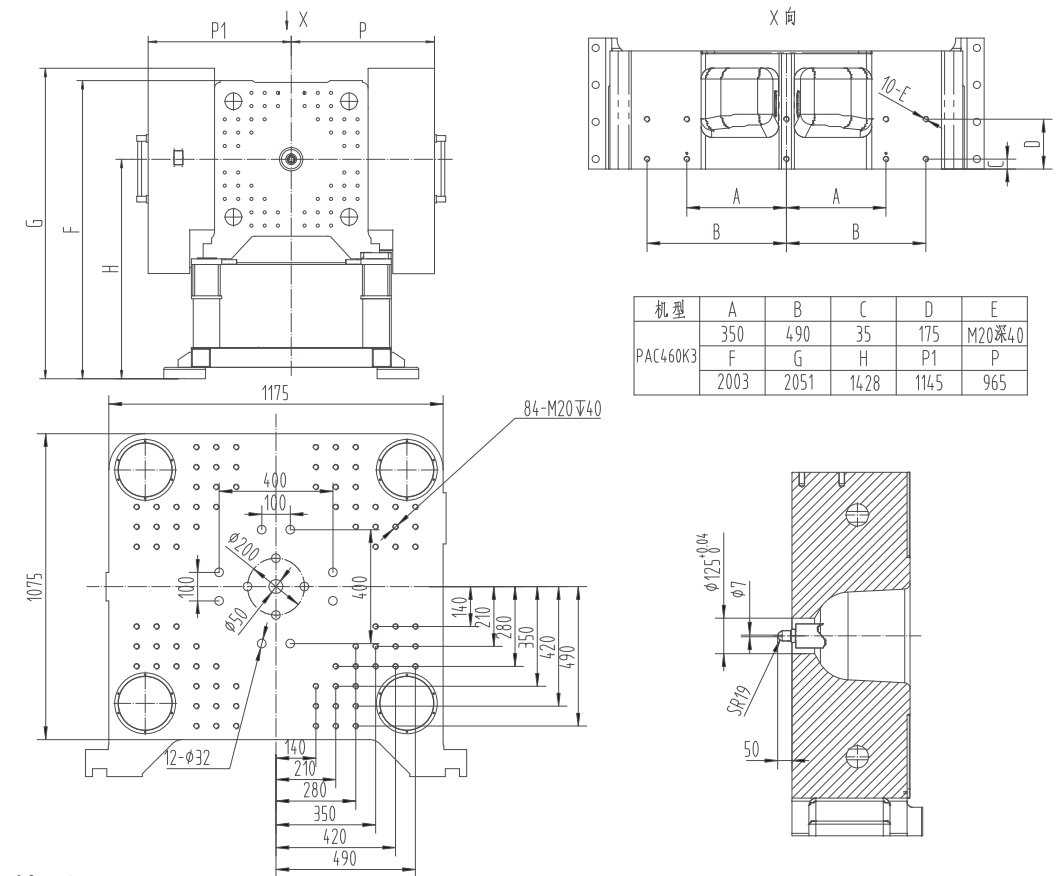
PAC460K3外形图
